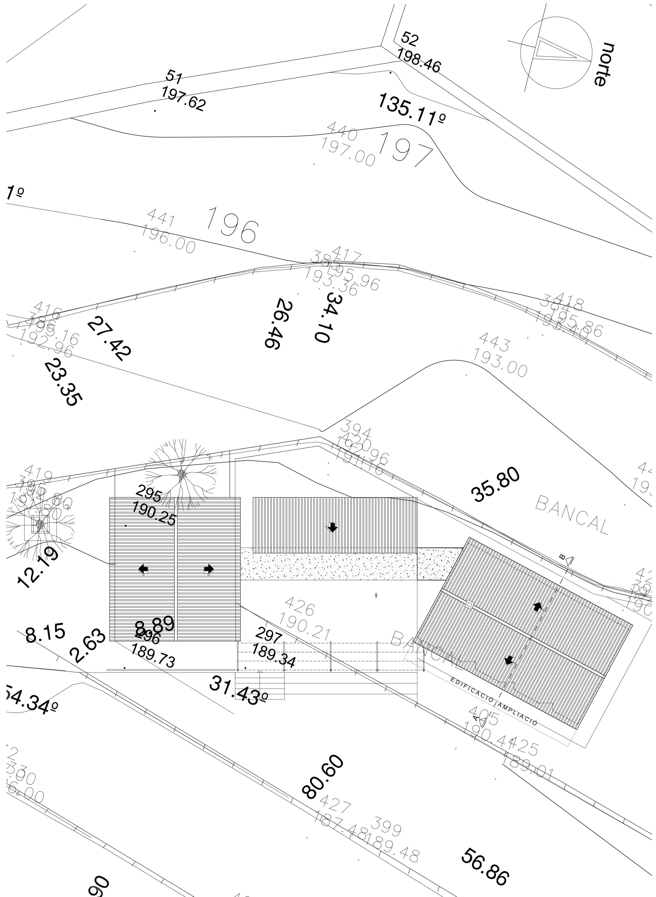
PLANTA COBERTES - SITUACIÓ A LA PARCEL·LA ESTAT FINAL ESCALA 1/100
